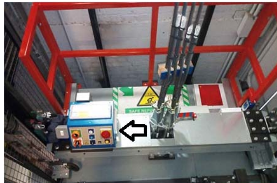
شکل ۶-۱۵- نمونه‌ای از تابلوی ریویزیون
