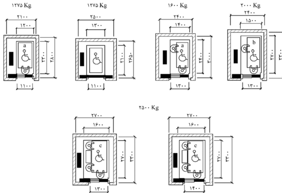
شکل ۵-۱۸- ایجاد چاهک برای آسانسور با کاربری عمومی
