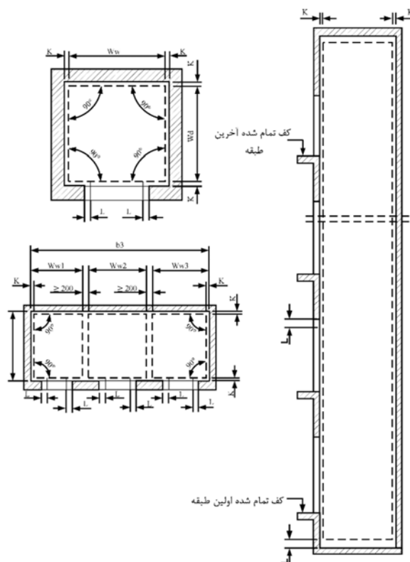
خطوط شاقولی و دیوارهای جداساز چاه‌های آسانسور
