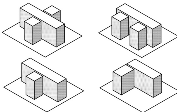
شکل ۷-۲ تقسیم ساختمان به قطعات مناسب با ایجاد درز انقطاع
