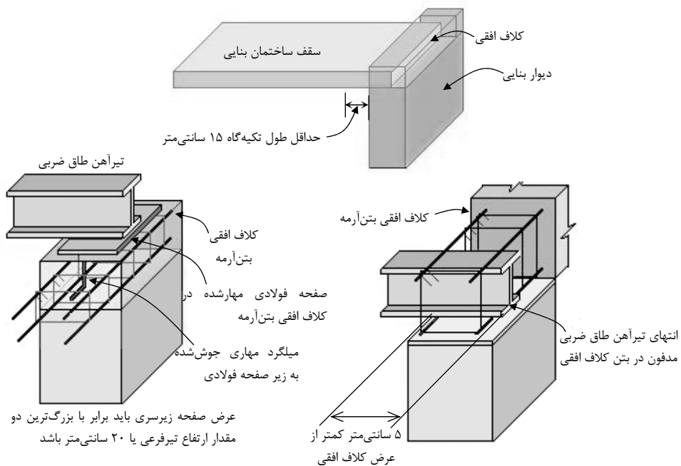
شکل ۲۶-۷ نمونه‌های اتصال تیرآهن سقف طاق ضربی به کلاف افقی بتن‌آرمه
